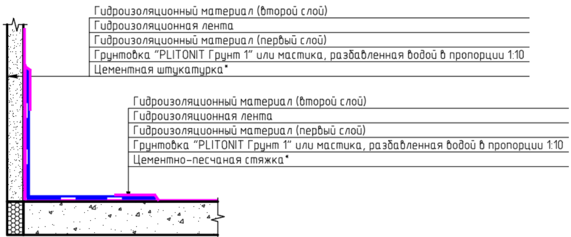
Разрез 1-1
